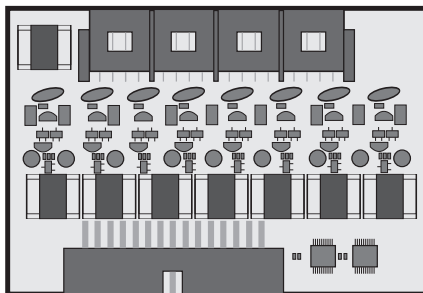
Placa de 08 ramais balanceados
