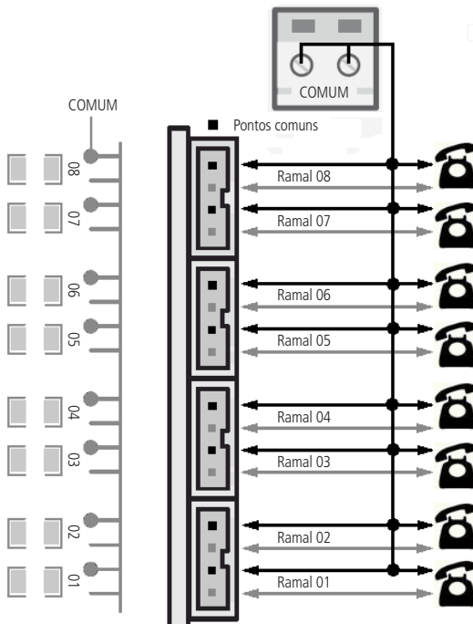
Ligação a partir de fio comum
