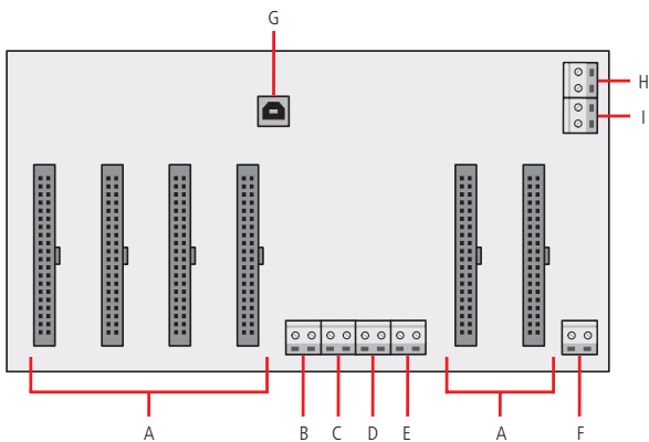
Placa base/CPU – COMUNIC 48
